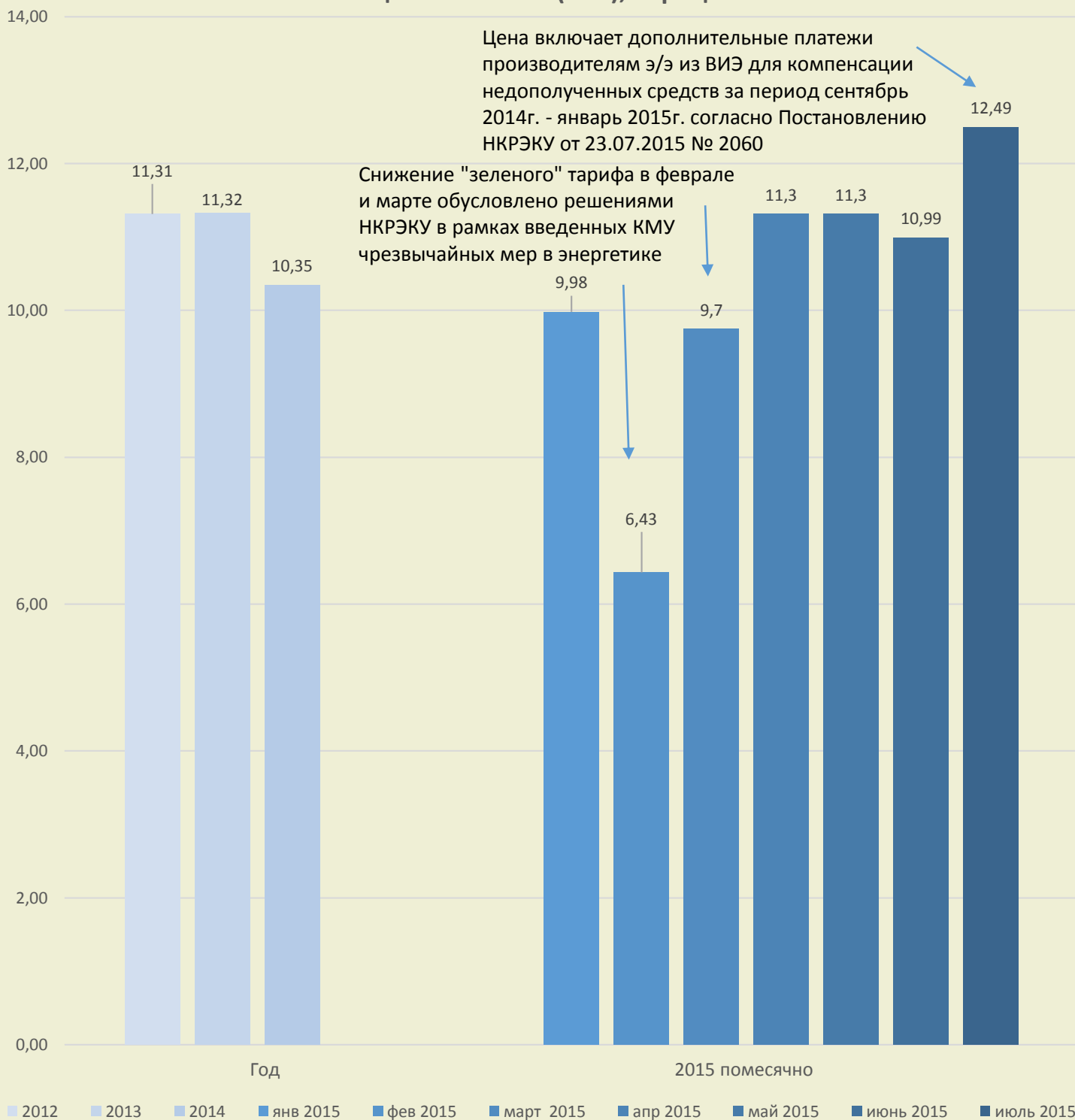
Фактическая цена за МВт*ч (ВЭС), евроцентов
