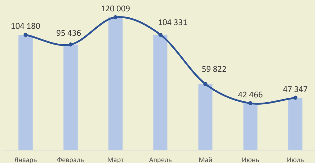
Фактический объем производства электрической энергии из энергии ветра (январь-июль 2015), тыс кВт·ч
