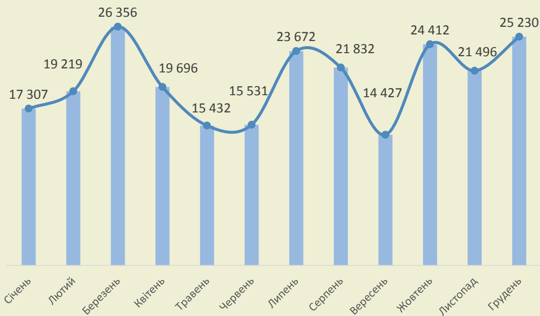
Фактичні обсяги виробництва електричної енергії з енергії вітру (2012 рік), тис кВт·год
