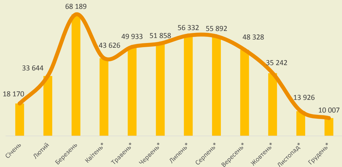
Фактичні обсяги виробництва електричної енергії з енергії сонячного випромінювання (2014 рік), тис кВт·год
