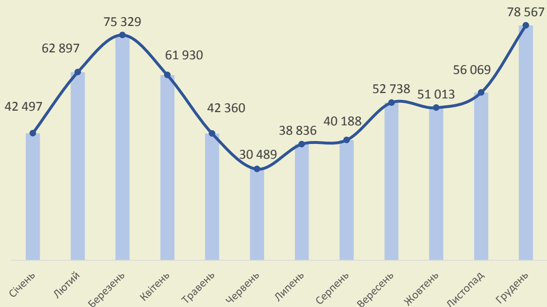
Фактичні обсяги виробництва електричної енергії з енергії вітру (2013 рік), тис кВт·год
