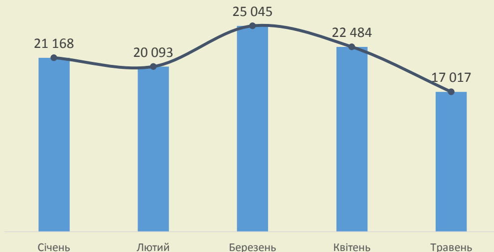
Фактичні обсяги виробництва електричної енергії МГЕС (січень-травень 2015), тис кВт·год
