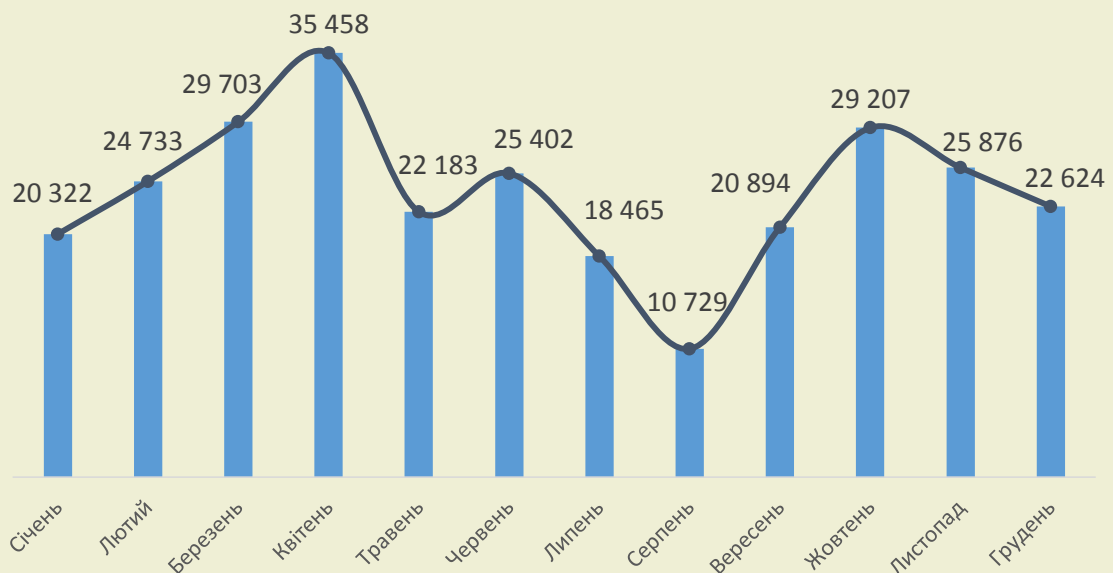
Фактичні обсяги виробництва електричної енергії МГЕС (2013 рік), тис кВт·год
