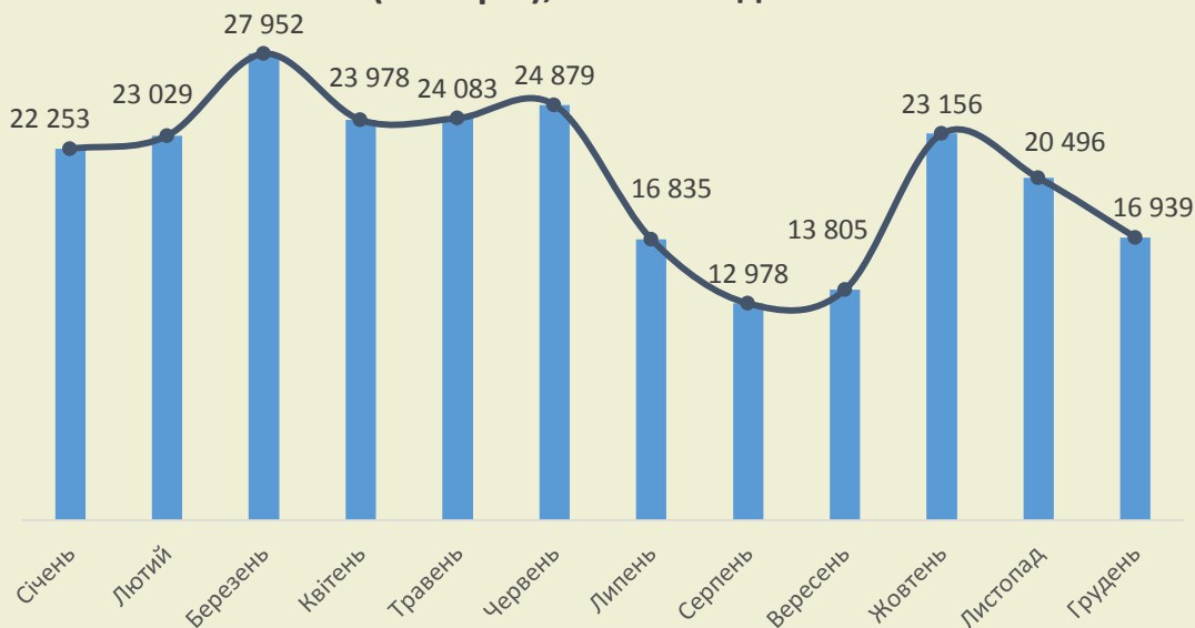
Фактичні обсяги виробництва електричної енергії МГЕС (2014 рік), тис кВт·год
