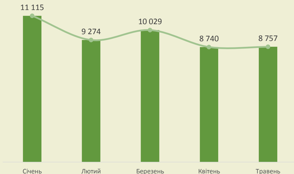
Фактичні обсяги виробництва електричної енергії з енергії біомаси (січень-травень 2015), тис кВт·год
