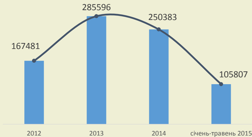
Фактичні обсяги виробництва електричної енергії МГЕС, тис кВт·год (2012 - 2015)
