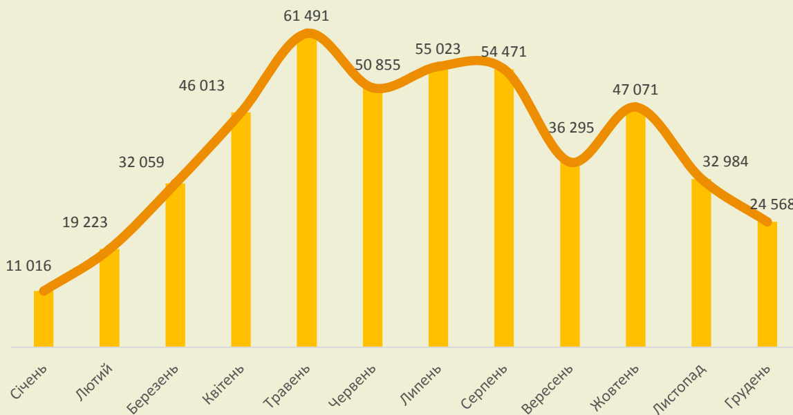
Фактичні обсяги виробництва електричної енергії з енергії сонячного випромінювання (2013 рік), тис кВт·год
