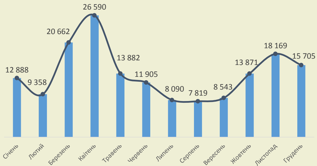
Фактичні обсяги виробництва електричної енергії МГЕС (2012 рік), тис кВт·год
